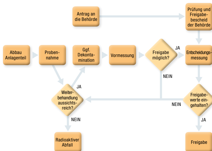
Abb. 34: Entscheidungsschema zur Freigabe von Anlagenteilen
